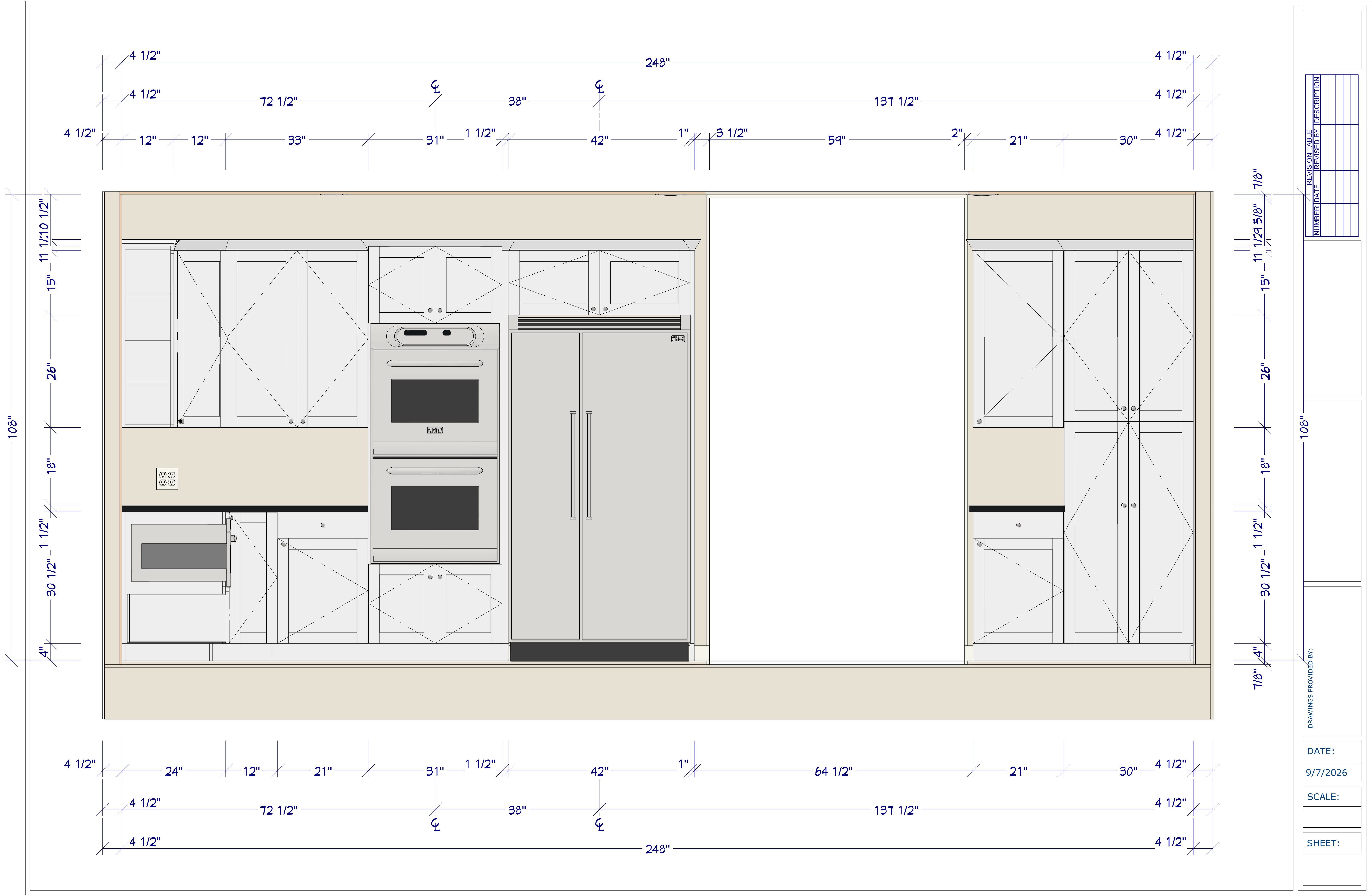
Elevation 2
